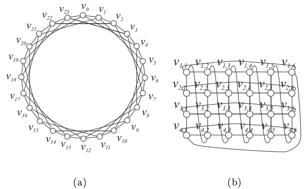
그림 1: 이중 루프 네트워크 G(24; 1, 4)
